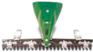
Doppelmesser-Mähbalken LASER
